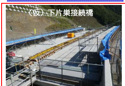
(仮)下片巣接続橋 橋桁上の床版コンクリート打設が終わり、壁高欄や中央分離帯などの構造物を作っています。
